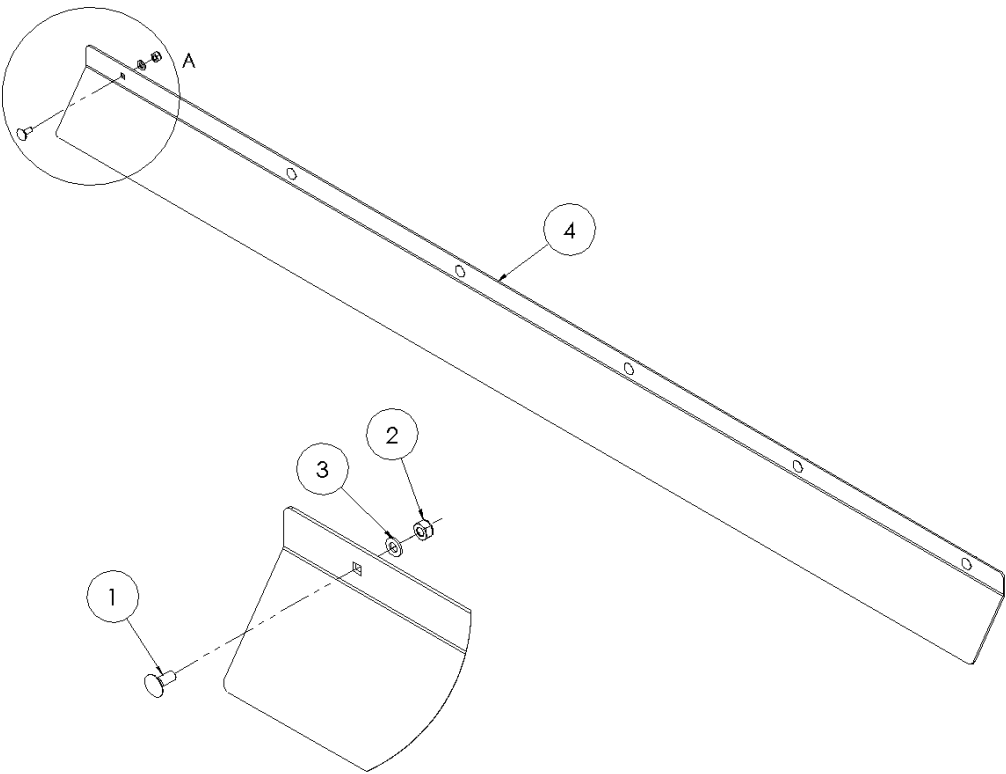
DETAIL A 1 : 5
