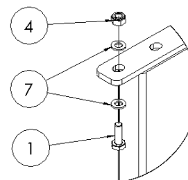
DETAIL B 1 : 5
