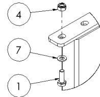
DETAIL A 1 : 5
