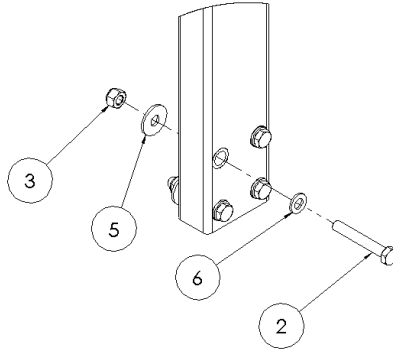
DETAIL B 1 : 5
