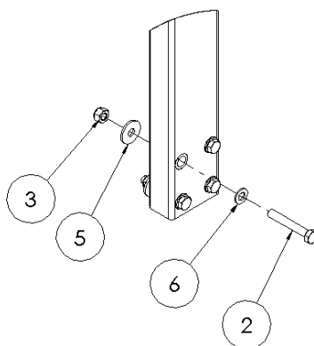
DETAIL A 1 : 7
